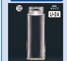
122 L-200ネジ瓶 53φ×H143(213ml) 60入 口部:47ネジ 材質ガラス
