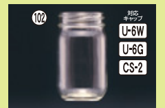
102 M-140瓶 55φ×H95(143ml) 100入 口部:51ネジ 材質ガラス
